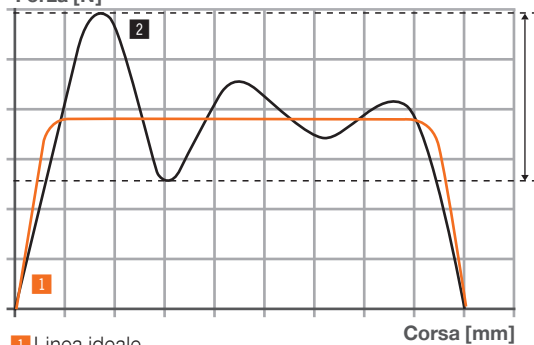
Forza [N]
