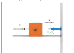
L6. Massa movimentata orizzontalmente con forza di azionamento ad accoppiamento geometrico
